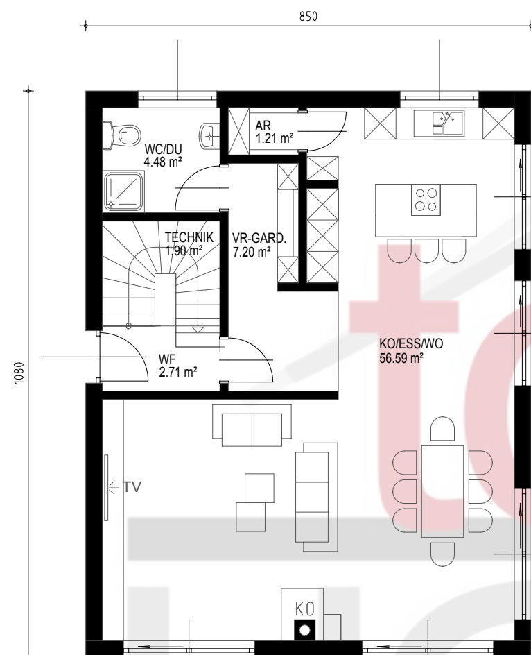
ERDGESCHOSS
